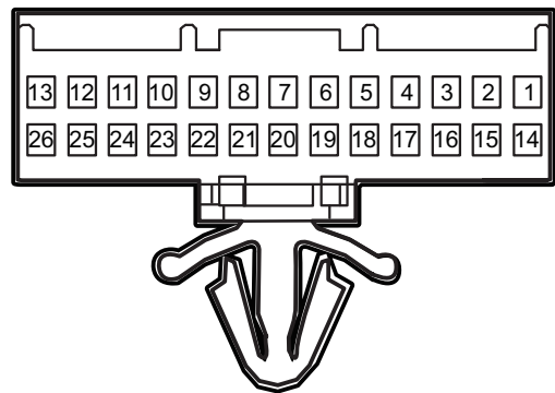
X03 底盘线束接仪表线束C（公端）
